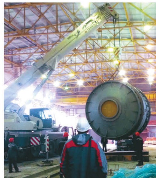
Филиал «Производство сплавов цветных металлов» АО «Уралэлектромедь». Монтаж короткобаранных плавильных печей (Италия).
